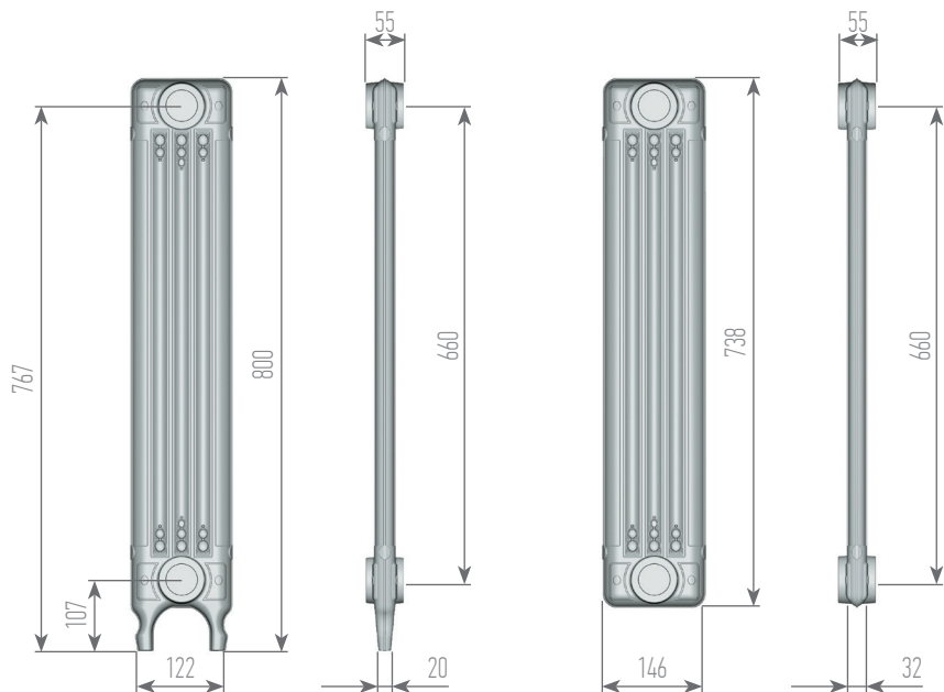
Размеры радиатора указаны без учета установленной арматуры и воздушного клапана
