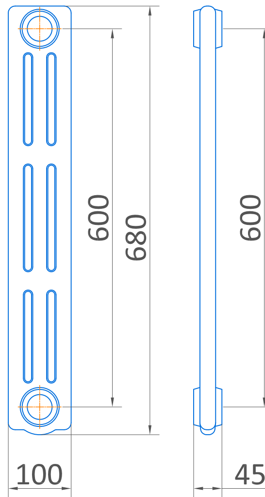
секция без ножек
