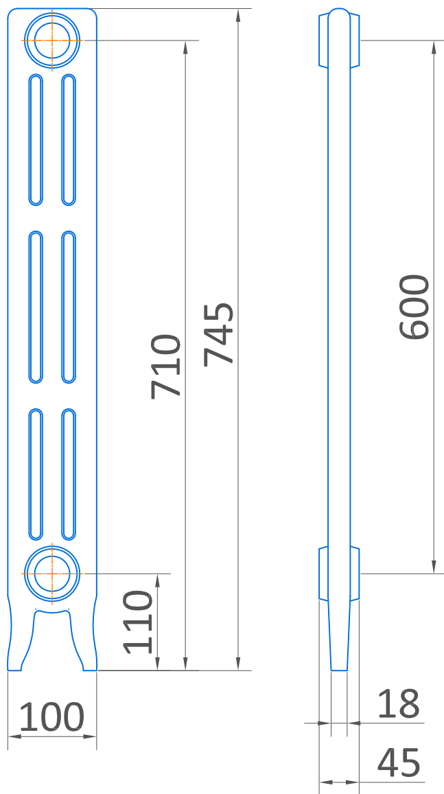
секция с ножками
