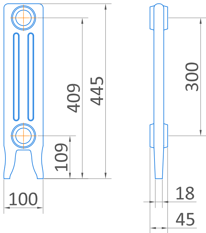
секция с ножками
