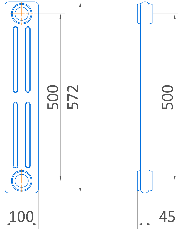
секция без ножек
