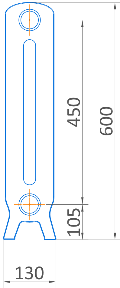
секция с ножками
