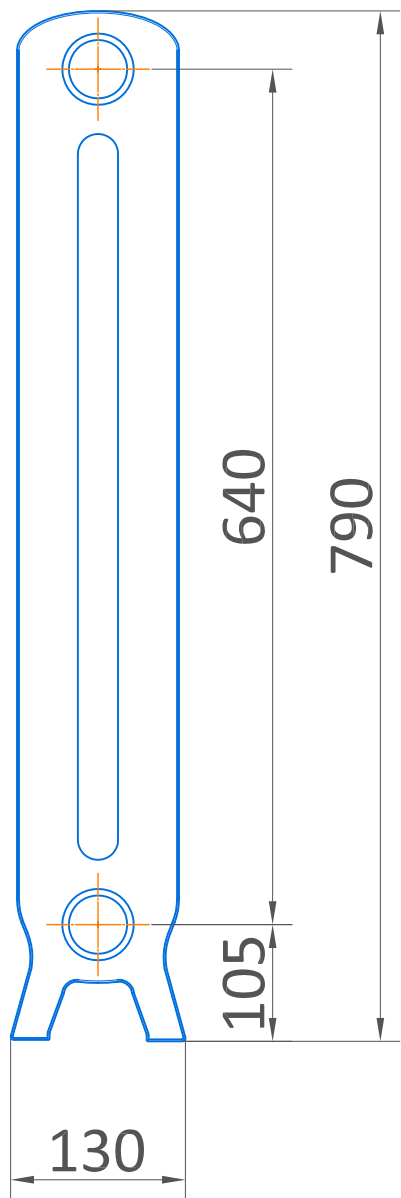
секция с ножками
